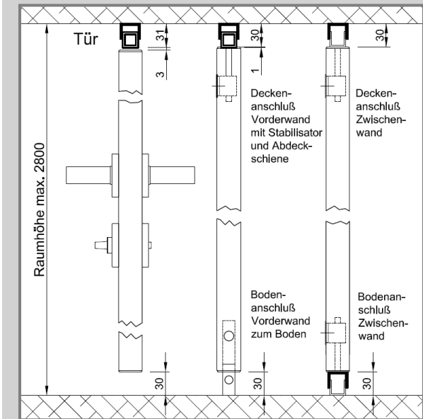
Systemskizze Höhenschnitt
